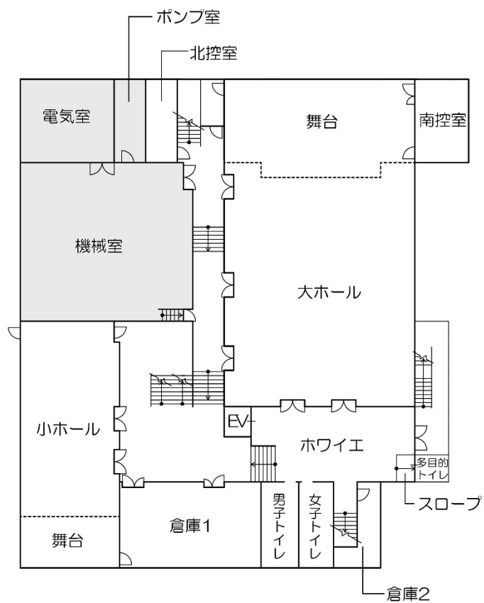
B1階平面図
