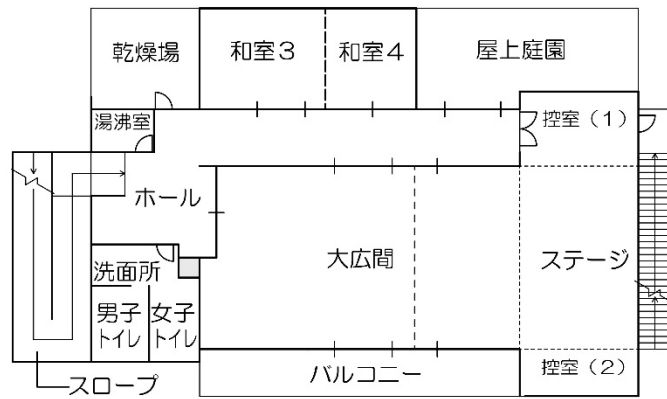
2階平面図
