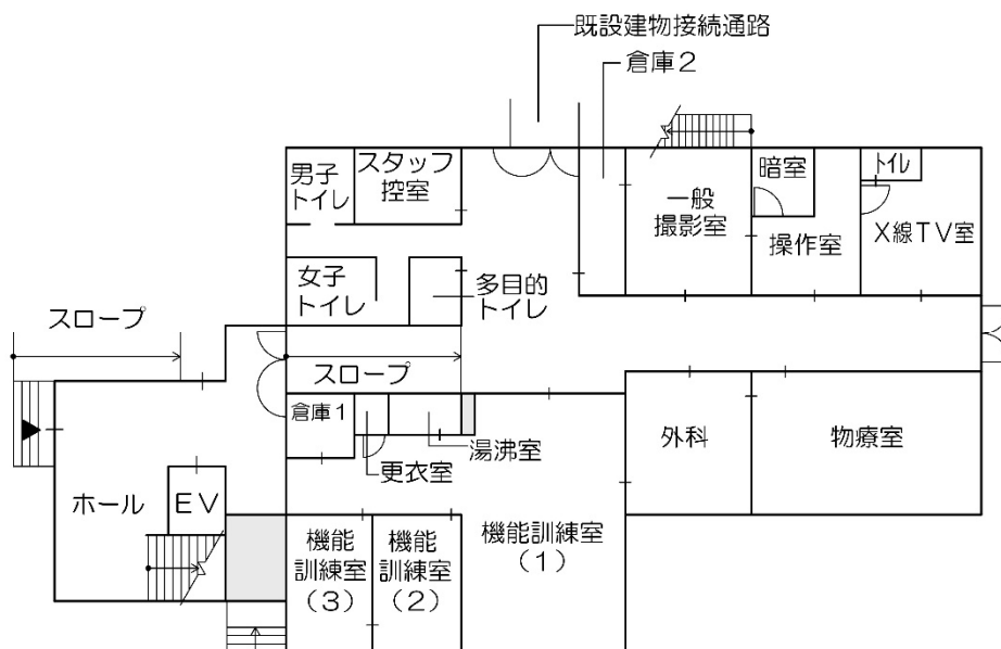
1階平面図
