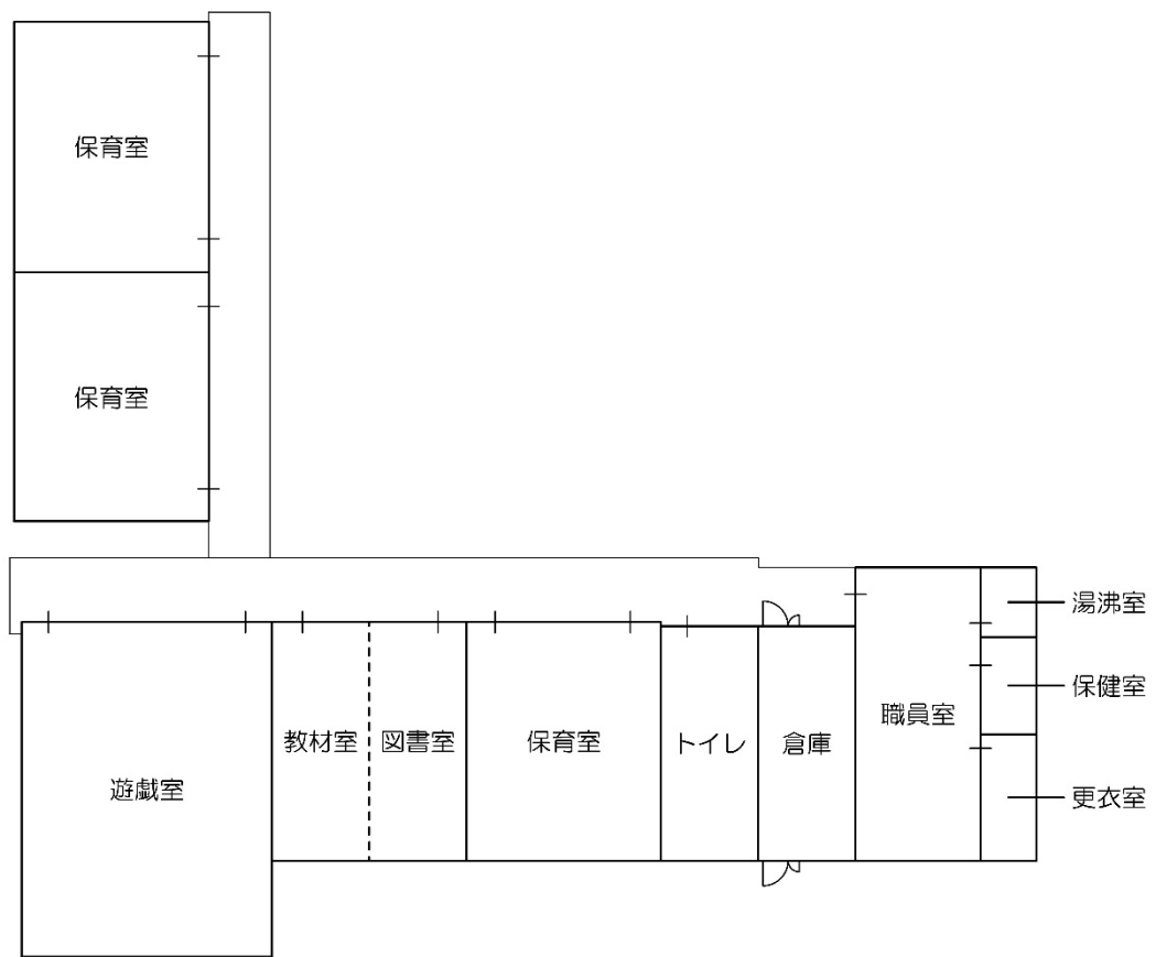
1階平面図
