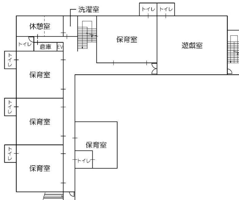
2階平面図
