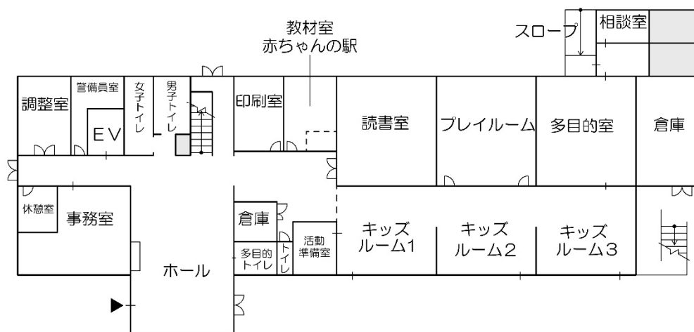
1階平面図
